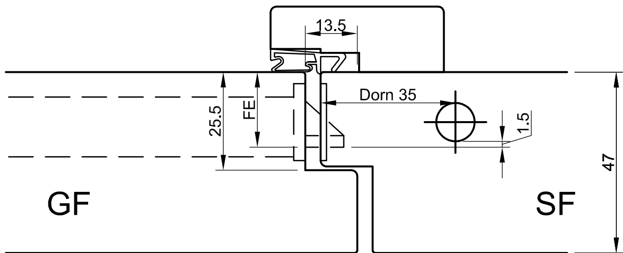
Falztreibriegel mit Gestänge nach oben und unten, automatik
